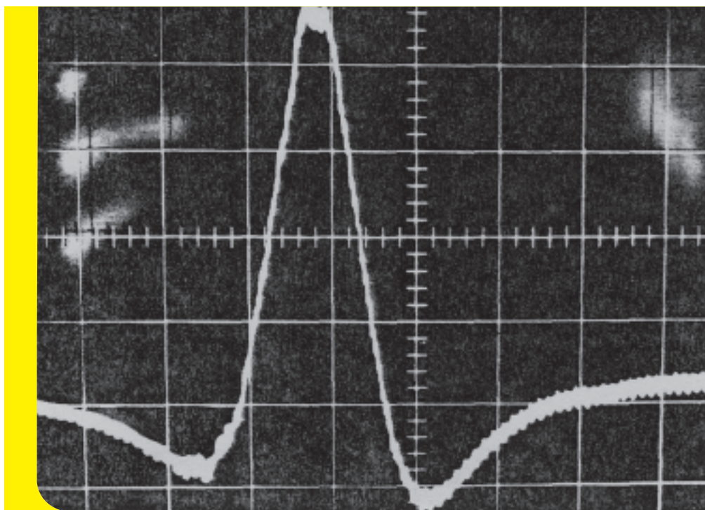
Illustration 26 : Fig. Champ électrique d'une nuée d'oiseaux de passage. On distingue le battement causé par les battements d'ailes collectifs sous la forme d'une interférence superposée, comme finement côtelée.
