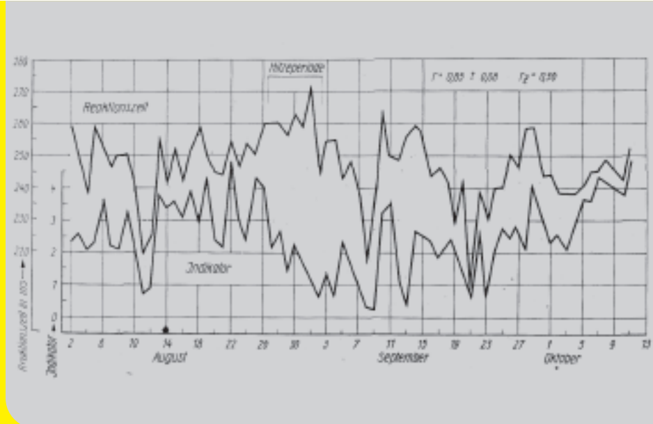
Illustration 5 La corrélation linéaire entre les activités des ondes infra longues électromagnétiques et le temps moyen de réaction chez les visiteurs d'une exposition n'est pas fortuite. Reiter, R. 1960 Meteorobiologie und Elektrizität der Atmosphäre. Akademische Verlagsges. Geest & Portig, Leipzig
